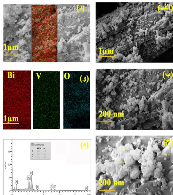
شکل ۵ - (الف - ج) تصویرهای FE-SEM، (د) تصویر FE-SEM مربوط به نقشه برداری عنصری، (و) نقشه توزیع عناصر و (ه) طیف EDS نمونه \text{BiVO}_4\text{-4h}
