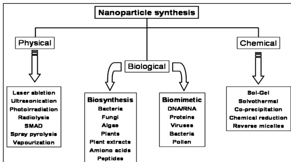
شکل ۱) نمای کلی از روش های مختلف فیزیکی، شیمیایی و بیولوژیکی ساخت نانوذرات [۶]
